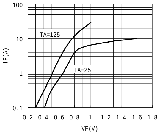
IF - VF
