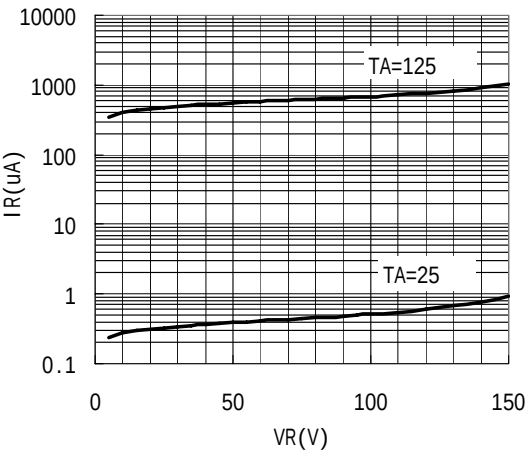
IR - VR
