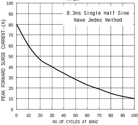
IFSM
