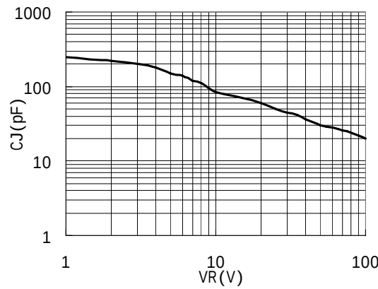
CJ - VR
